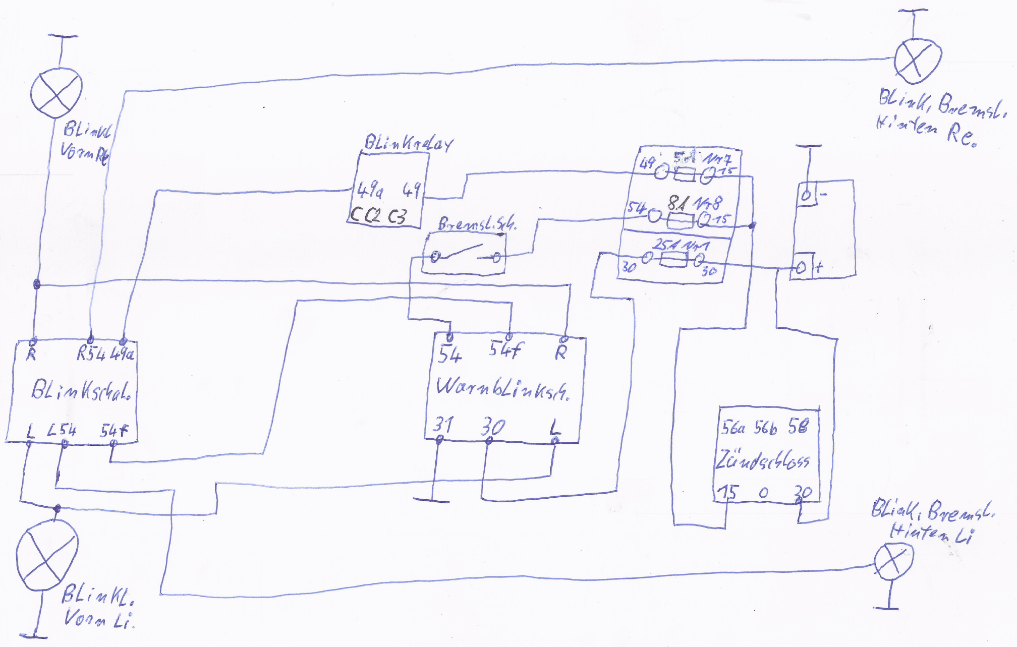
Zweikreis Blinkanlage hinten Blinker + Bremse in einem
